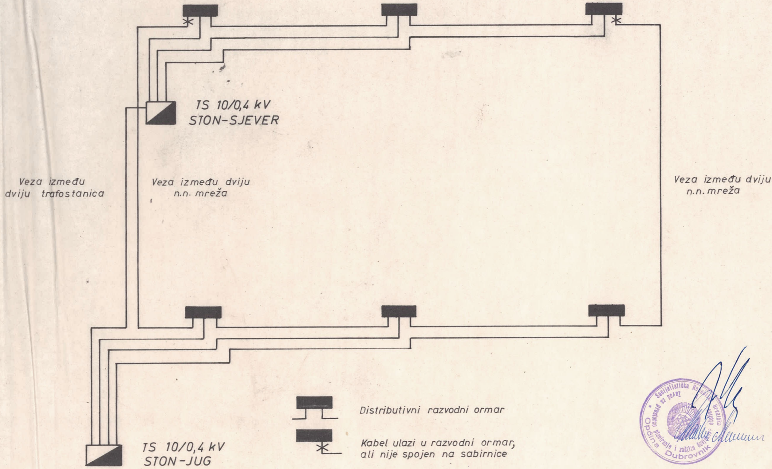
BLOK-SHEMA razvoda glavnih niskonaponskih vodova u užem dijelu stare gradske jezgre
