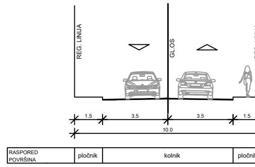
POPREČNI PRESJEK "B"
