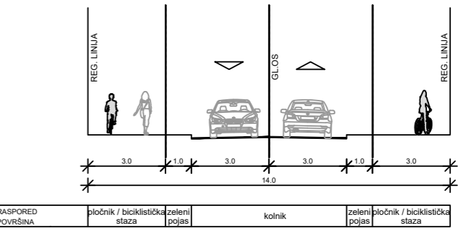
POPREČNI PRESJEK "A"
