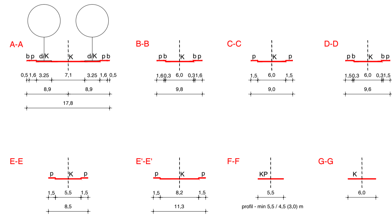
KARAKTERISTIČNI POPREČNI PRESJECI ULICA MJ 1:500 K - kolnik, KP - kolno-pješačka prometnica, P - parking, p - pješačka staza, d - dvorod
