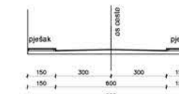
KARAKTERISTIČAN POPREČNI PRESJEK C - C
