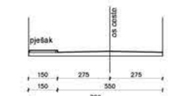
KARAKTERISTIČAN POPREČNI PRESJEK D - D
