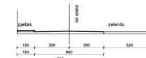
KARAKTERISTIČAN POPREČNI PRESJEK F - F
