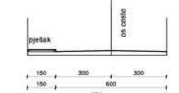
KARAKTERISTIČAN POPREČNI PRESJEK G - G
