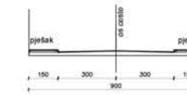
KARAKTERISTIČAN POPREČNI PRESJEK B - B
