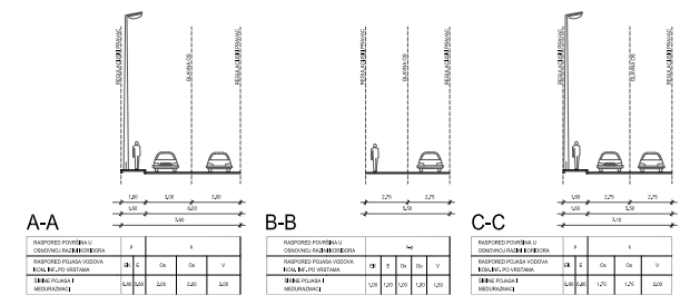
Poprečni presjek ulice s načelnim rasporedom pojaseva komunalne infrastrukture
