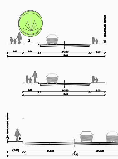
POPREČNI PRESJECI CESTA GLAVNA GRADSKA ULICA mjerilo 1:100
