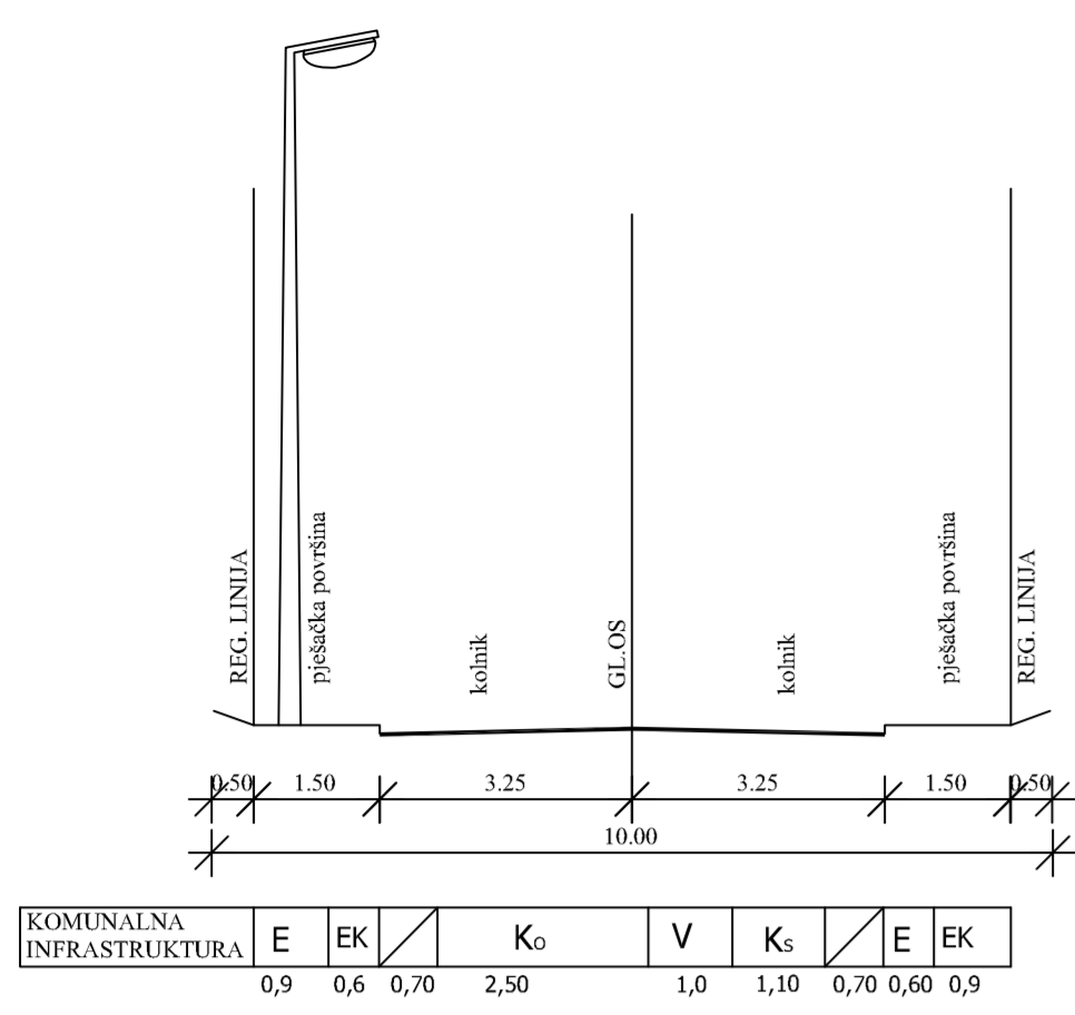
POPREČNI PRESJEK "1"
