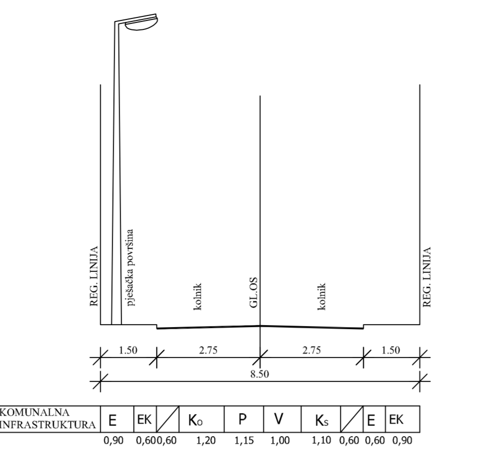
POPREČNI PRESJEK "3"
