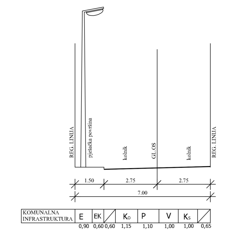
POPREČNI PRESJEK "5"
