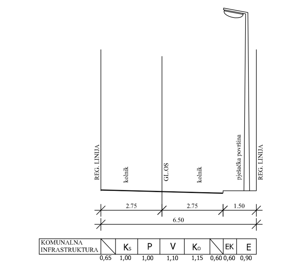
POPREČNI PRESJEK "7"
