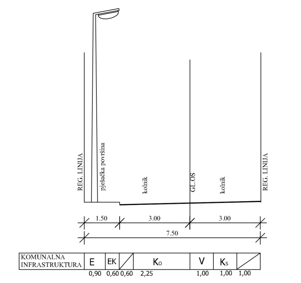
POPREČNI PRESJEK "6"
