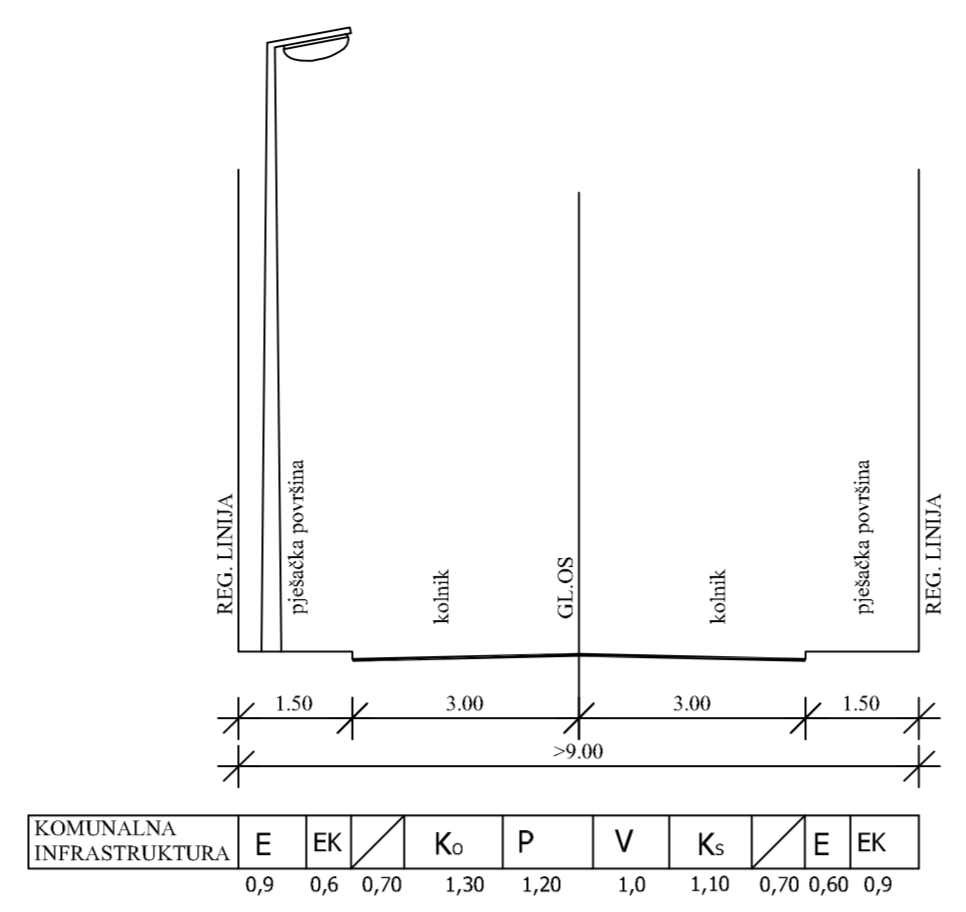
POPREČNI PRESJEK "4"
