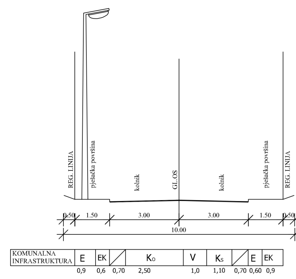
POPREČNI PRESJEK "2"
