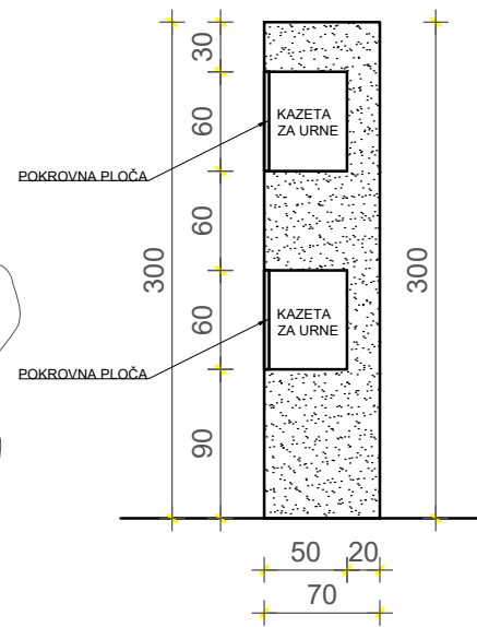
PRESJEK 2-2
