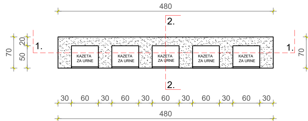
TLOCRT
