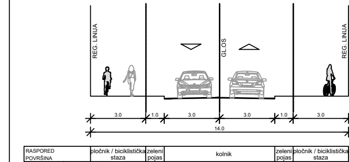
POPREČNI PRESJEK "A"
